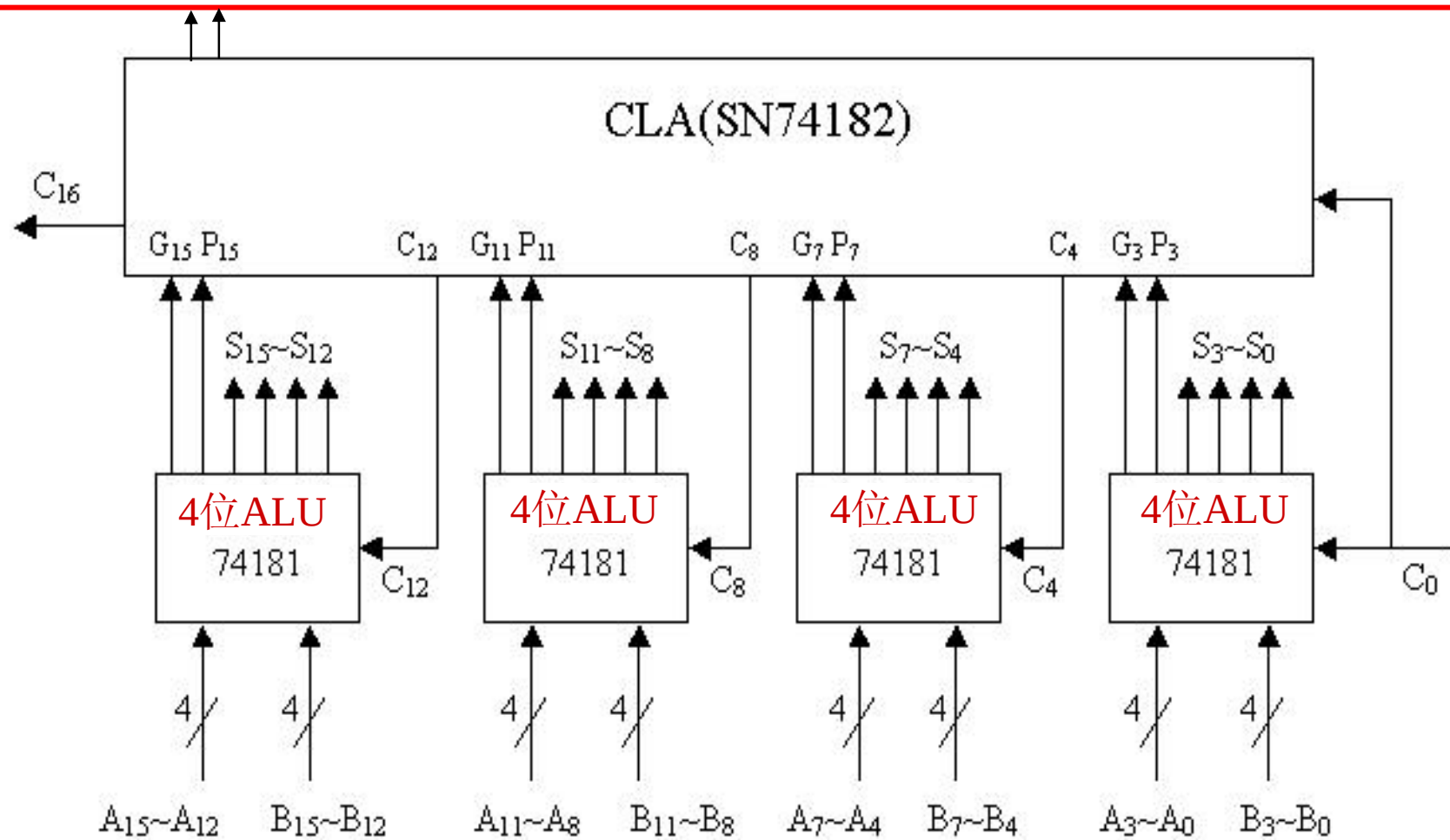
16位两级先行进位ALU
