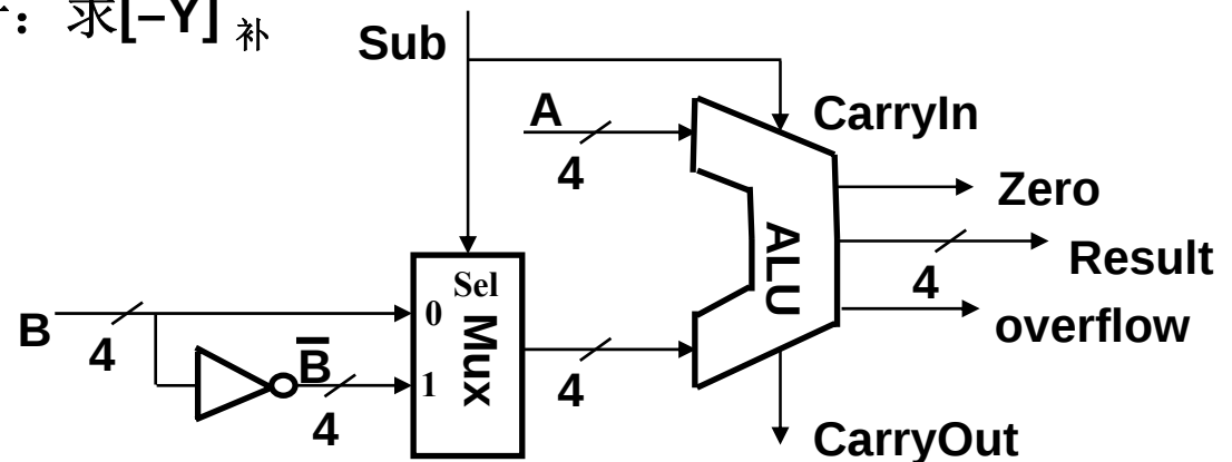
补码加减运算部件
